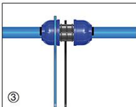
Umístění montážního klíče na spojovacím prstenci a na tělu spoje (Positioning of spanners on coupling ring and fitting body)
